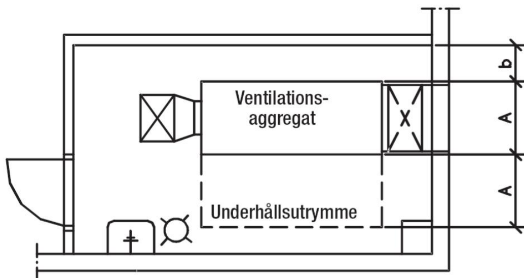
Figur 4. Placering av underhållsutrymme för inkapslat ventilationsaggregat och dimensioneringsexempel. A är ventilationsaggregatets bredd och b är 0,4 gånger ventilationsaggregatets höjd eller minst 400 mm.
