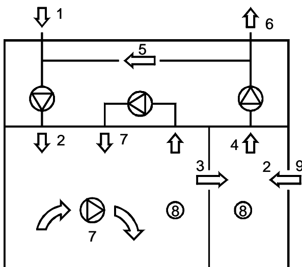
Figur 1. Benämningar på luftströmmar: 1. Uteluft, 2. Tilluft, 3. Överluft, 4. Frånluft, 5. Återluft, 6. Avluft, 7. Cirkulationsluft, 8. Inneluft, 9. Uteluft (ersättande luft).
