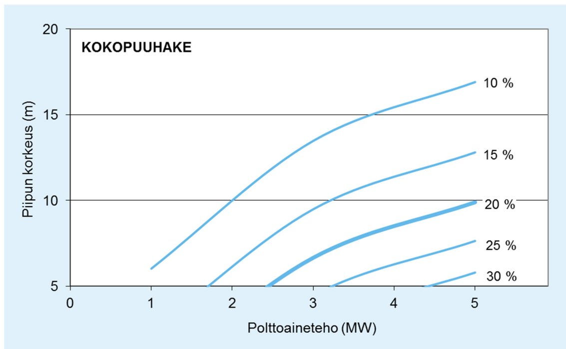
Kuva 12. Kokopuuhaketta käyttävien 1–5 MW kokoisten energiantuotantoyksiköiden piipun korkeuden mitoitus suhteessa pienhiukkasten vuorokausiohjeeseen verrannolliseen pitoisuuteen (% ohjeavosta). Vähimmäispiipunkorkeus (piipun suuaukon korkeus metreinä maanpinnasta) on aina vähintään 5 metriä. Lisäksi piipunkorkeuden tulee olla vähintään 1,5 kertaa laitosrakennuksen korkeus.
