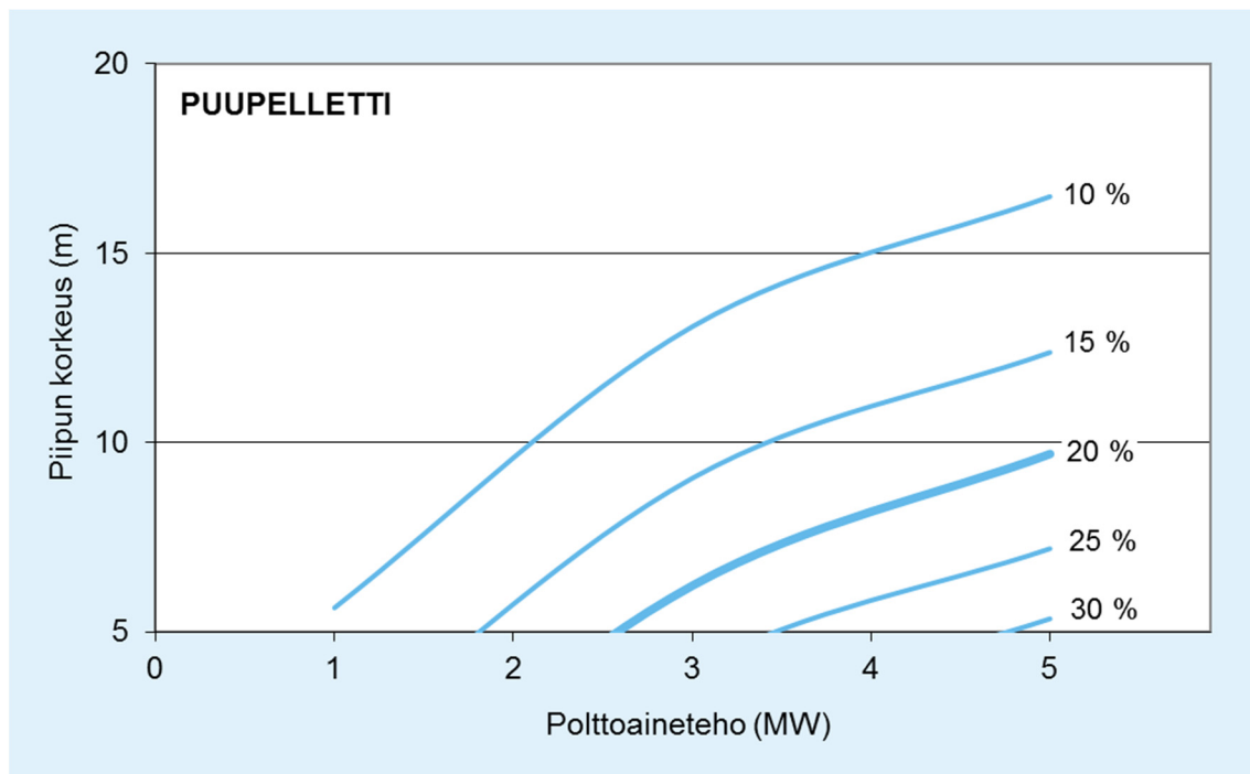
Kuva 11. Puupellettejä käyttävien 1–5 MW kokoisten energiantuotantoyksiköiden piipun korkeuden mitoitus suhteessa pienhiukkasten vuorokausiohjeeseen verrannolliseen pitoisuuteen (% ohjeavosta). Vähimmäispiipunkorkeus (piipun suuaukon korkeus metreinä maanpinnasta) on aina vähintään 5 metriä. Lisäksi piipunkorkeuden tulee olla vähintään 1,5 kertaa laitosrakennuksen korkeus.
