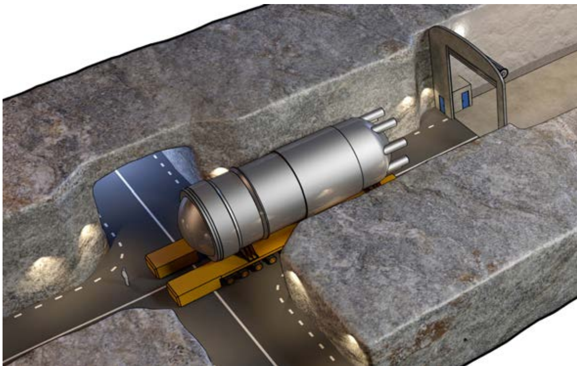
Figur 7-12. Illustration av två fordon av typen SPMT som kopplats ihop.
