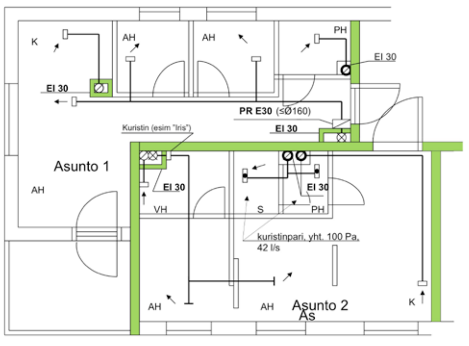
Kaavio 16 Esimerkki asuinrakennuksen asuntojen liittymisestä keskusilmanvaihtolaitteistoon, kun konehuone on palvelemiensa tilojen yläpuolella.
