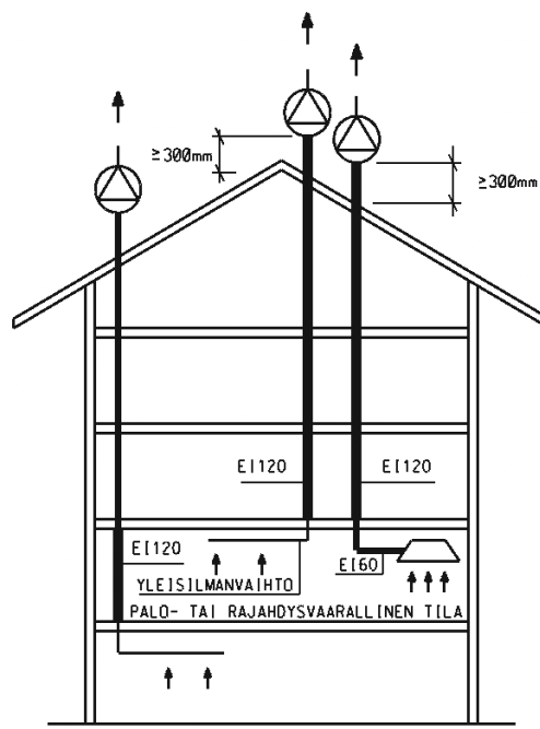
Kuva 2 Palo- ja räjähdysvaarallisen tilan ilmakanavien palonkestävyys.
