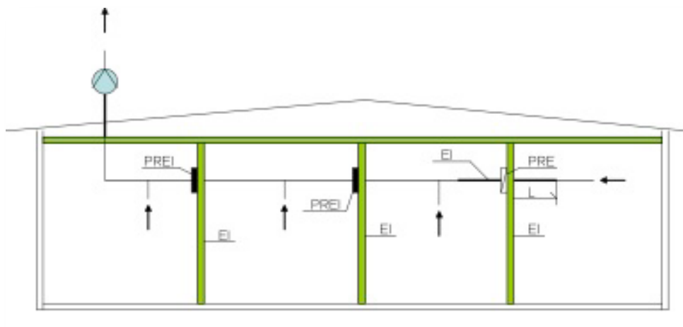
Kaavio 7 Esimerkki E7-ohjeen mukaisesta palonrajoittimen käytöstä palo-osaston rajalla tavanomaisia tiloja käsittävässä rakennuksessa.
