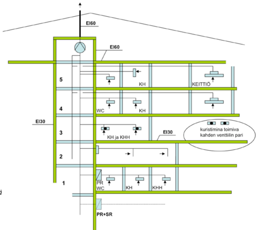
Kaavio 15 Esimerkki asuinkerrostalon keskitetystä keskusilmanvaihtolaitteistosta, jonka konehuone on palvelimiensa tilojen yläpuolella.
