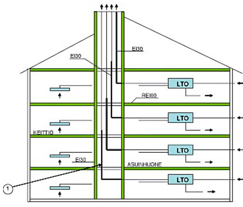
Kaavio 14 Asuntokohtainen ilmanvaihtolaitteisto asuinkerrostalossa. Jäteilmakanavat johdetaan erillisinä vesikatolle. Jäteilma- kanava paloeristetään kerroskorkeuden verran, pystysuoralta osaltaan vähin- tään 2,5 m:n matkalta (1) ja kannakoi- daan huolellisesti. Huomioitava myös jäteilmakanavan kondenssieristys
