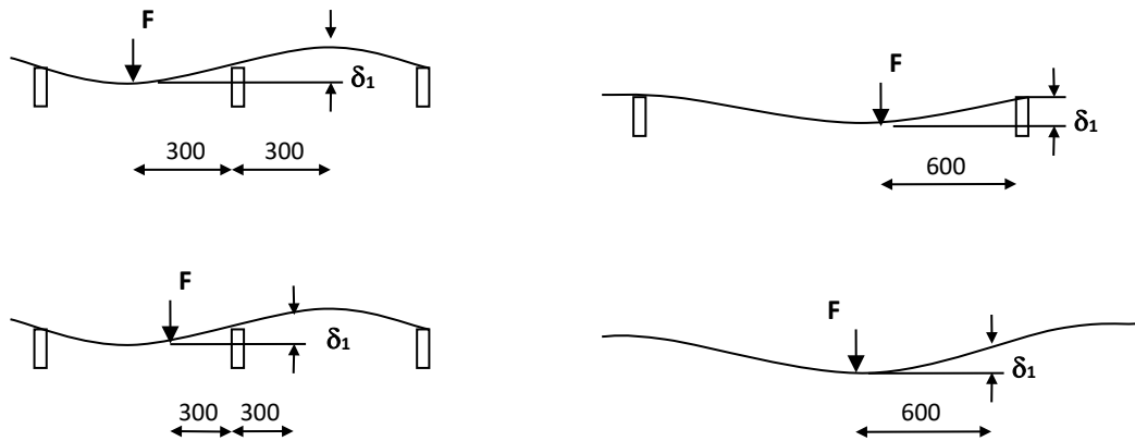
Bild 2. Exempel på nedböjning av golvet ytkonstruktion
