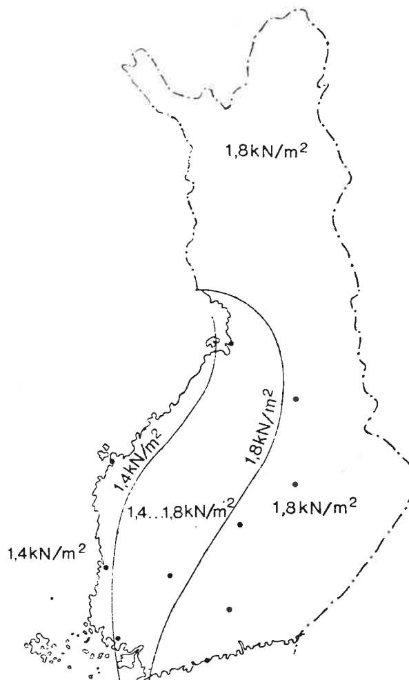
Kuva 1 Kattojen lumikuormat
