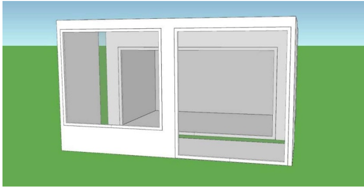
Kuva 8. Simulaatiossa käytetty parvekemalli. Parvekkeen keskellä on 285 mm leveä pilari. Puolet parvekekaiteesta on valoa läpäisemätöntä materiaalia ( h=700 mm) ja puolet lasitettua kaidetta. Parvekkeen syvyys 2000 mm. Kuvakaappaus simulaatio-ohjelmasta.
