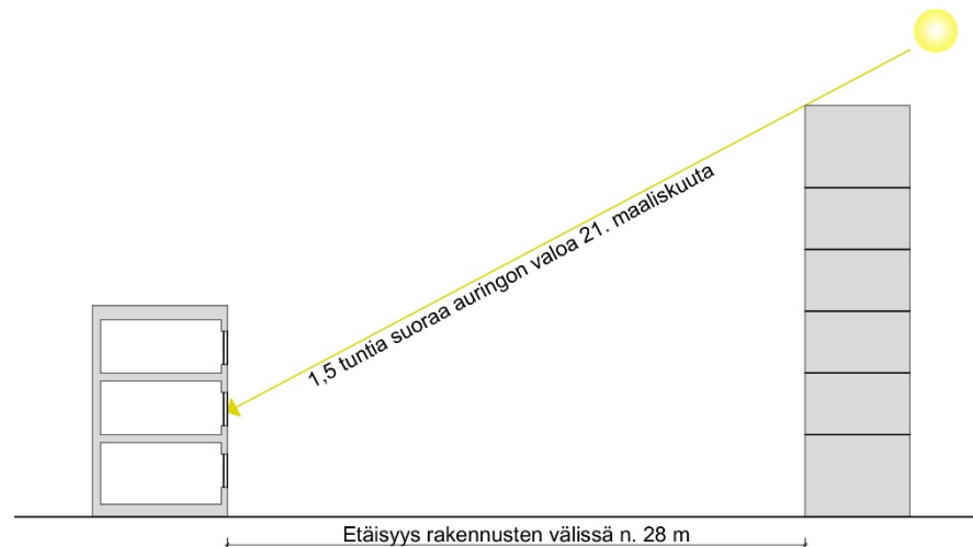
Kuva 23. Etäisyys toisen kerroksen etelään avautuvan asunnon ja sitä vastapäätä olevan kuusikerroksisen pitkän rakennusmassan välissä tulisi olla noin 28 metriä Helsingissä, jotta standardin vaatimus 1,5 tunnin suorasta auringonpaisteesta 21. maaliskuuta täyttyisi.
