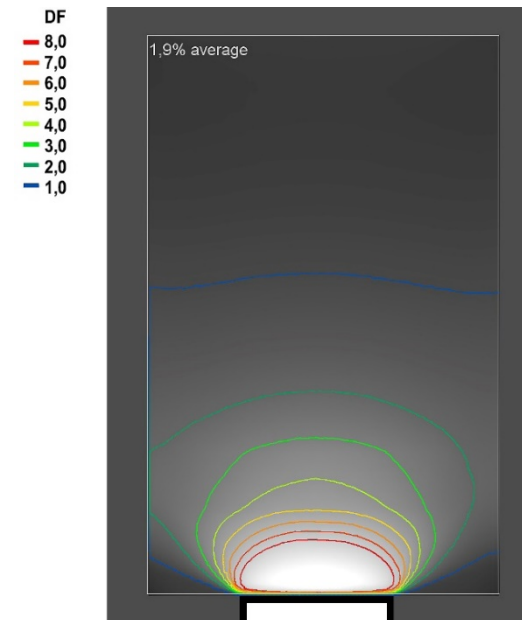
Kuva 12. Keskimääräinen päivänvalosuhde ja päivänvalosuhteen ääri viivat.
