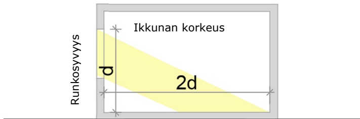
Kuva 10. Nyrrkisääntönä on pidetty, että huoneen pystyy valaisemaan tyydyttävästi päivänvalolla syvyyteen, joka on kaksinkertainen ikkunan yläreunan korkoon.
