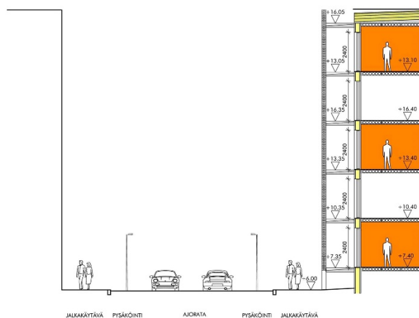
Kuva 7. Leikkaus kadun poikki. Väri osoittaa tarkasteltavat asunnot.
