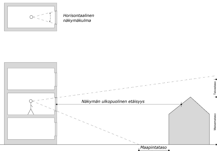
Kuva 22. Standardissa määritellyt kriteerit näkymälle.
