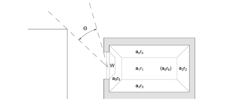
Kuva 13. Keskimääräisen päivänvalosuhteen laskukaava.
