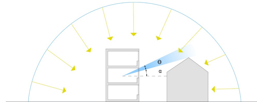
Kuva 6. \theta = taivaskulma, kuvastaa näkyvää taivasta \alpha = estetty kulma, kuvastaa ulkoista estettä (esim. vastapäinen rakennus)
