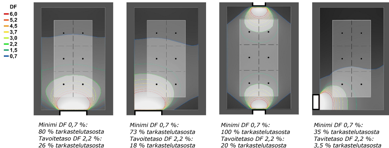
Kuva 9. Standardin EN 17037:2018 mukaan päivänvalosuhte (DF) tulisi olla Helsingissä 0,7 % melkein koko tarkastelutasolla (95 %) ja saavuttaakseen keskitasoisen päivänvalaistuksen tulisi DF olla 2,2 % puolessa (50 %) tilan tarkastelutasoa. Jopa täysin esteettömällä näkymällä on vaikea saavuttaa näitä ehtoja Suomen 10 % ikkunapinta-alasäännöllä. Pelkästään ikkunan sijoittelu vaikuttaa tilan valaistukseen.
