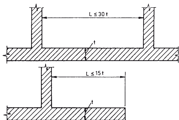
Kuva 8. Seinän tuenta.
