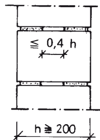
b) rakosauma
