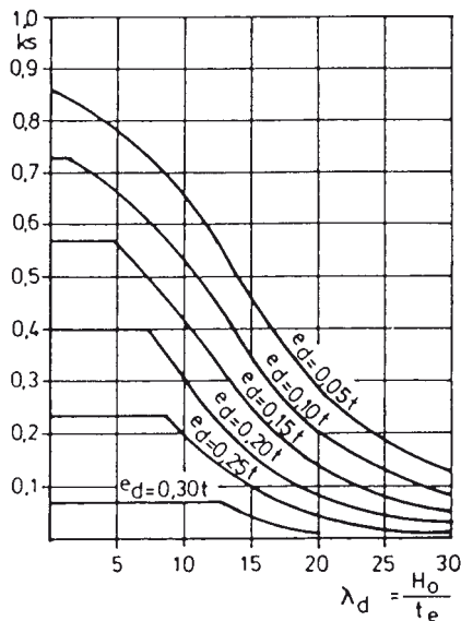
Kuva 6. Kerroin k_s .
